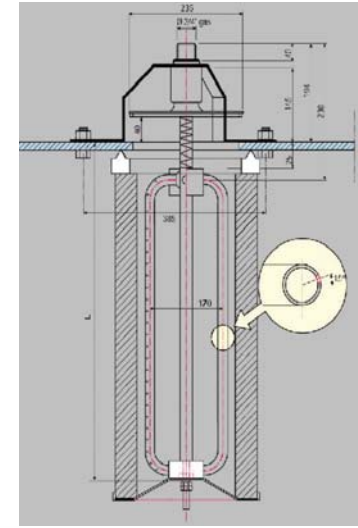
Filters mit automatisch programmierter Reinigung (Rotojet)
