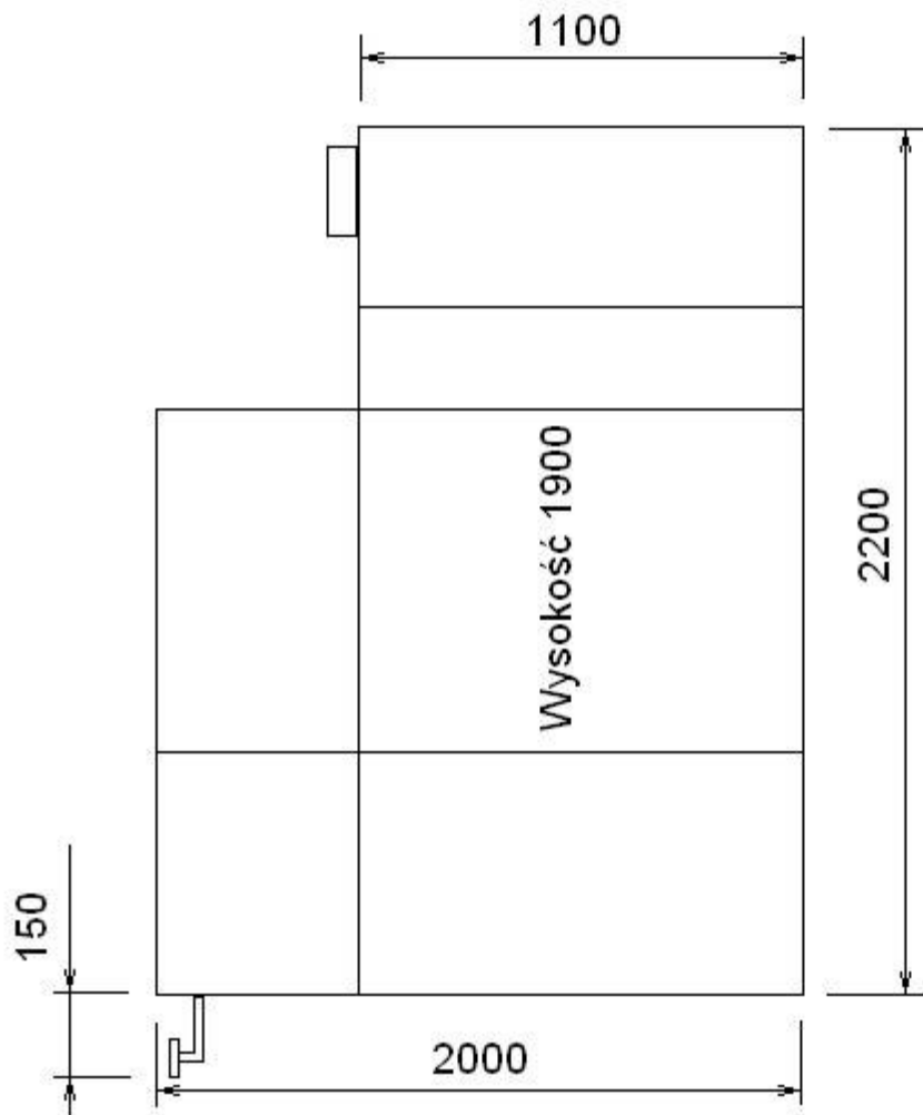
Trawiarka alkaliczna, moduł II
