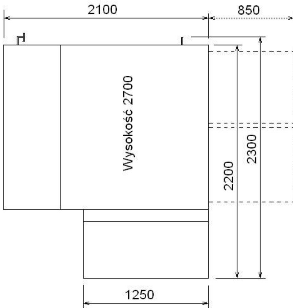
Trawiarka alkaliczna, moduł I
