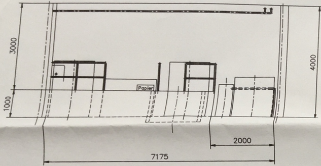
Schnitt A-A
