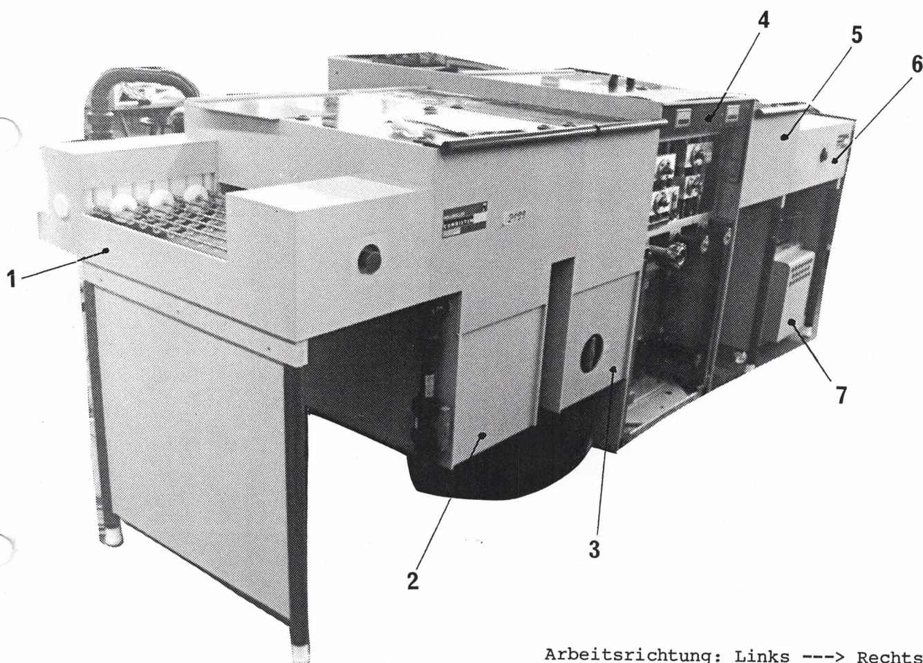
Illustr. 484.02: Bürstlinie A 2199 - Bedienseite
